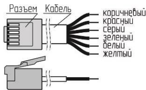
Вилка на кабель TR6P6C (нумерация проводов)
