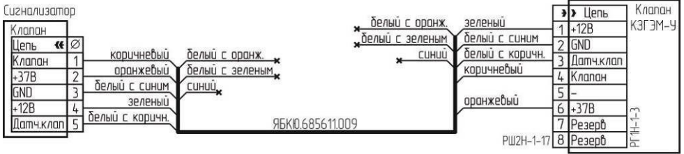
Рисунок В.3 – Схема подключения клапана КЗГЭМ-У с разъемом PSH-1-3.
