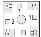
Рисунок В.6 – Схема подключения клапана КЗЭУГ с разъемом TJ1A-6P6C
