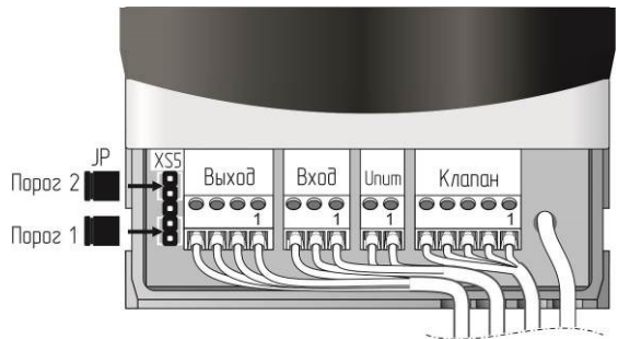
Рисунок 4 – Расположение разъемов
