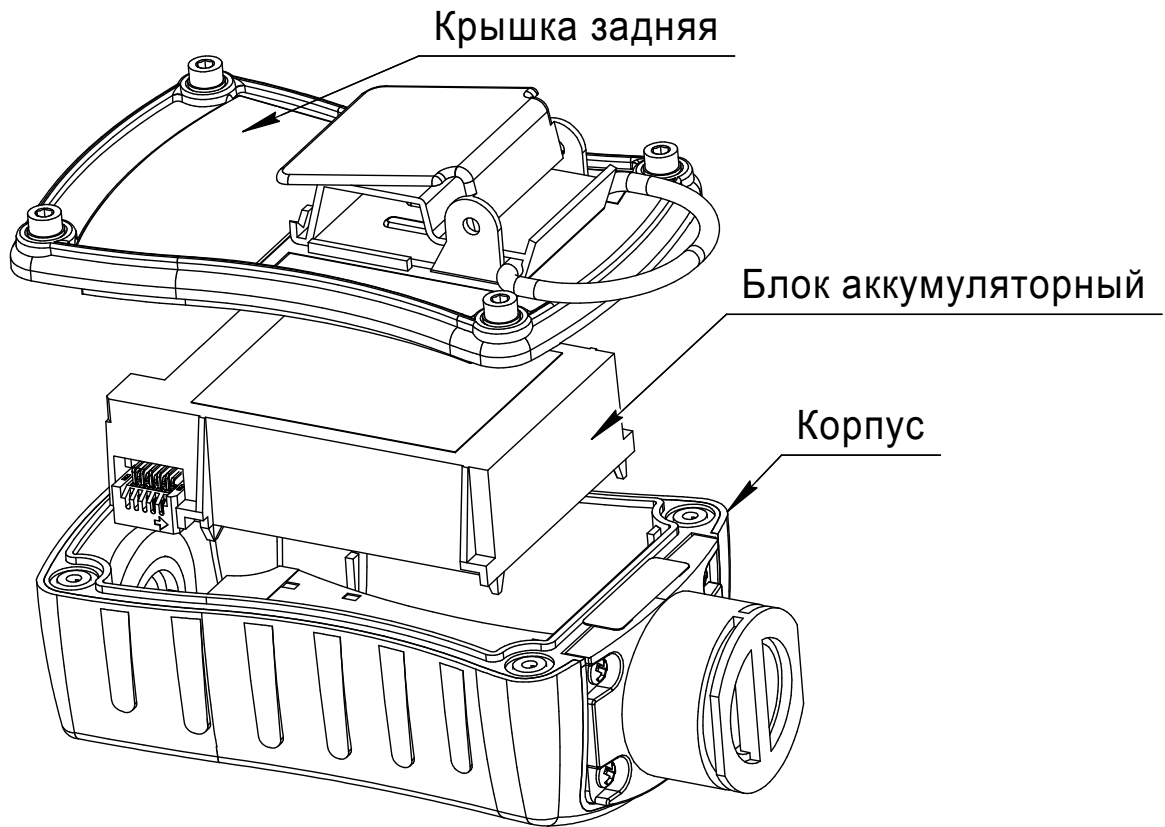
Рисунок 4.1 – Схема установки/замены блока аккумуляторного
