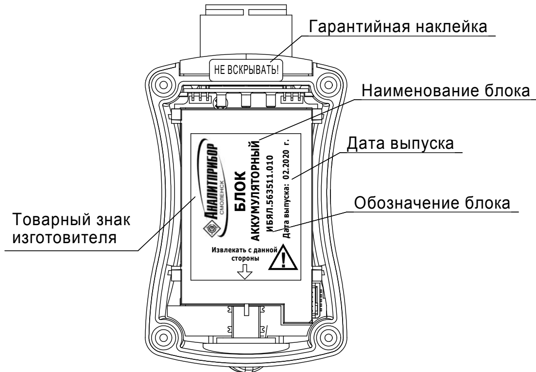
Рисунок 1.6 – Маркировка аккумуляторного блока и расположение гарантийной (пломбирочной) наклейки
