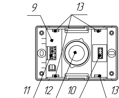
Рисунок 1.1 - Сигнализаторы оксида углерода и горючих газов СТГ-1. Внешний вид
