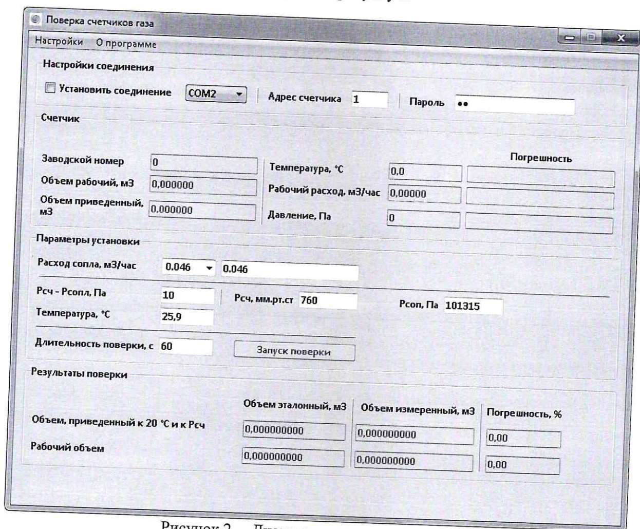
Рисунок 2 – Диалоговое окно программы «FlowP»
